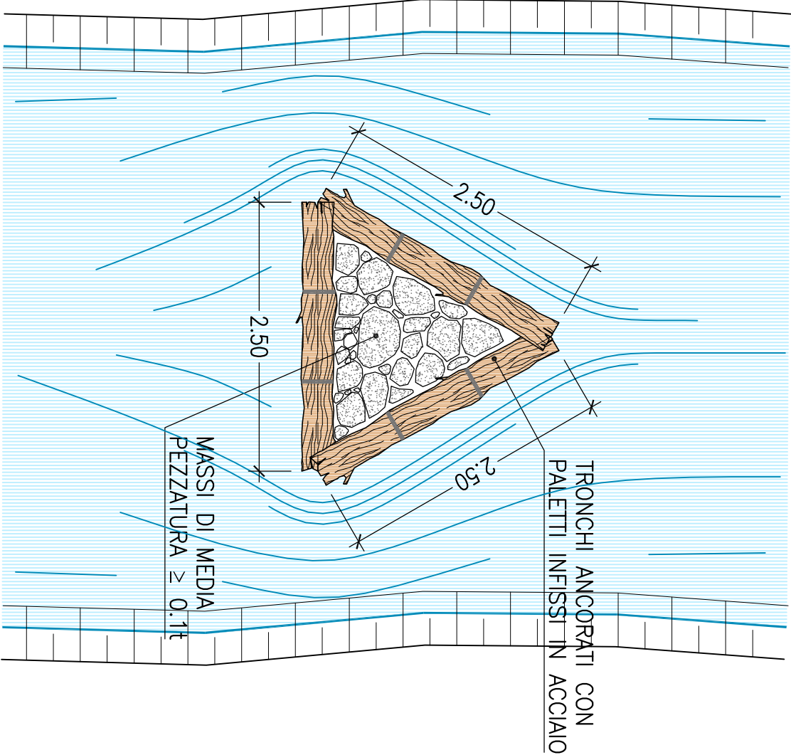
DEFFLETTORE A "V" IN ASSE ALVEO IN TRONCHI E MASSI scala 1:50
