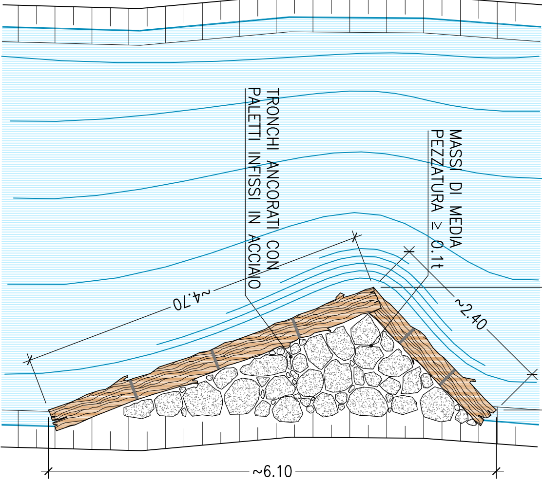
DEFFLETTORE IN TRONCHI E MASSI scala 1:50
